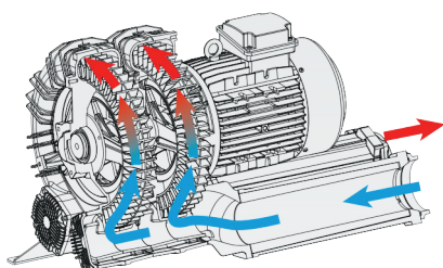
Serie: TS Girante gemellare Monostadio
