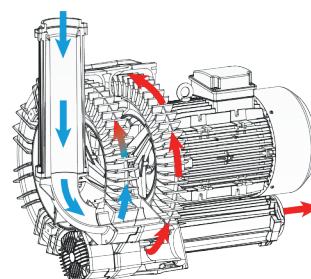
Serie: TD Girante gemellare Doppio stadio
